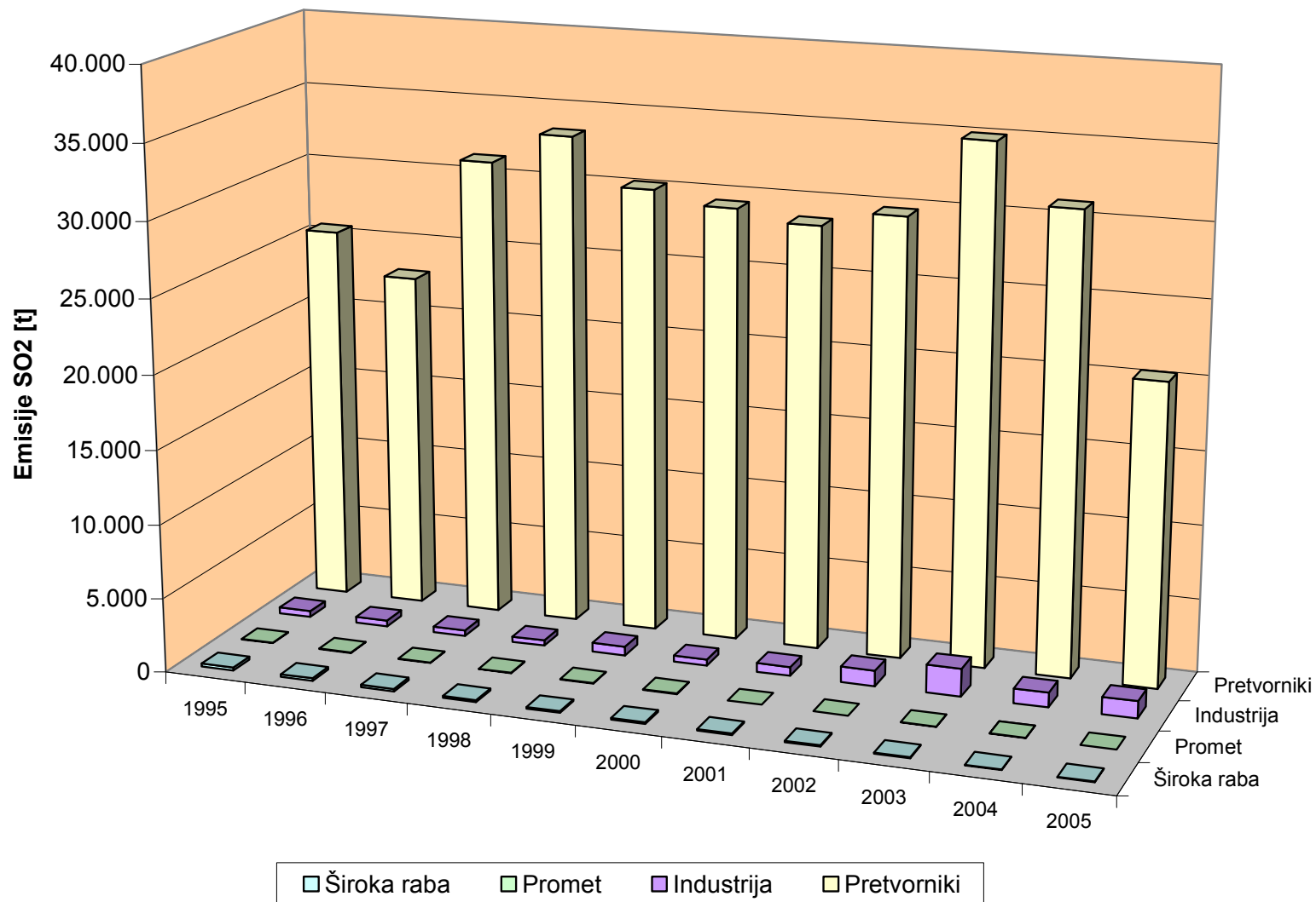
Slika P1.1: Ocena emisij SO 2 v Zasavju v obdobju 1995-2005.
