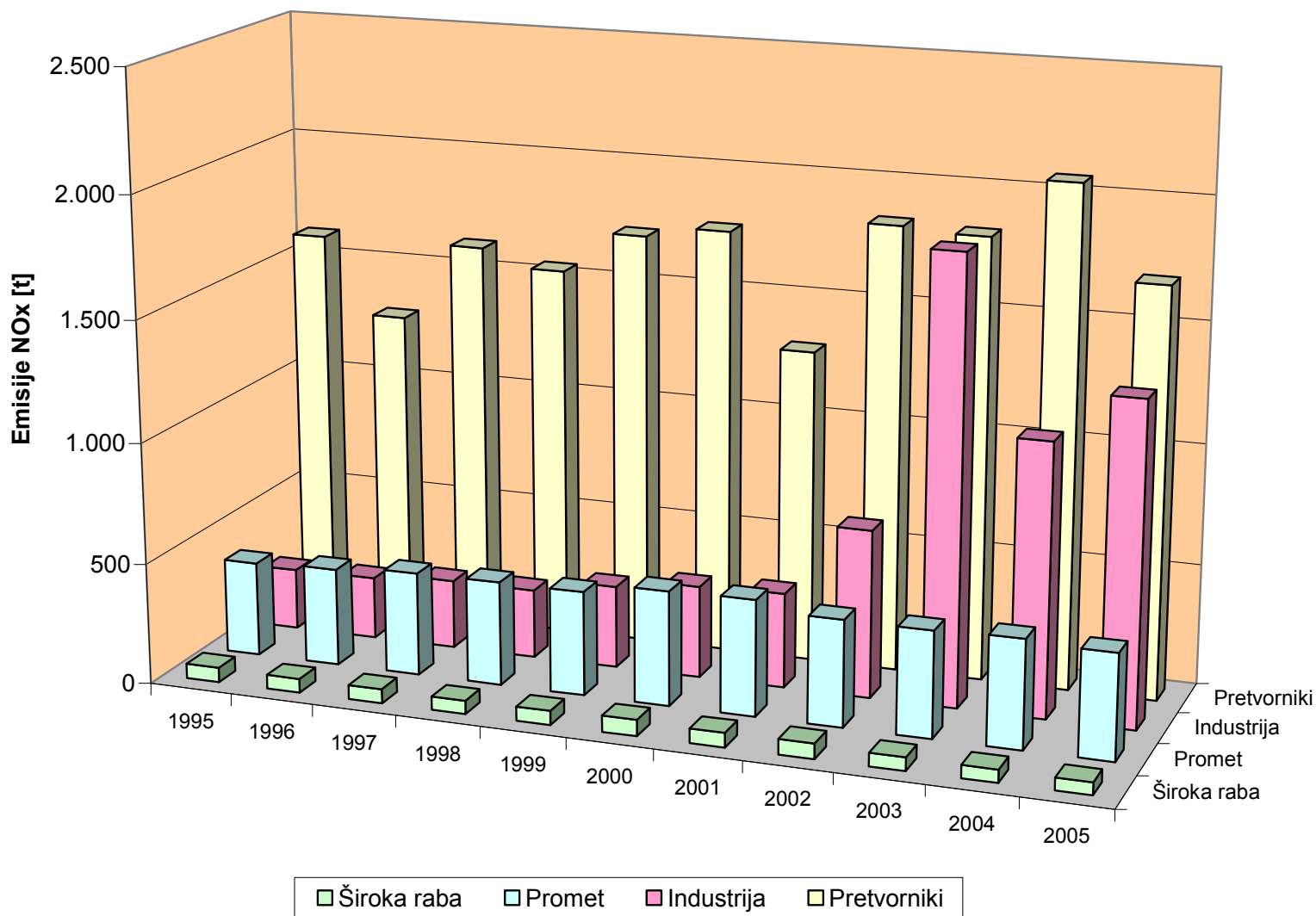
Slika P1.2: Ocena emisij NO x v Zasavju v obdobju 1995-2005.
