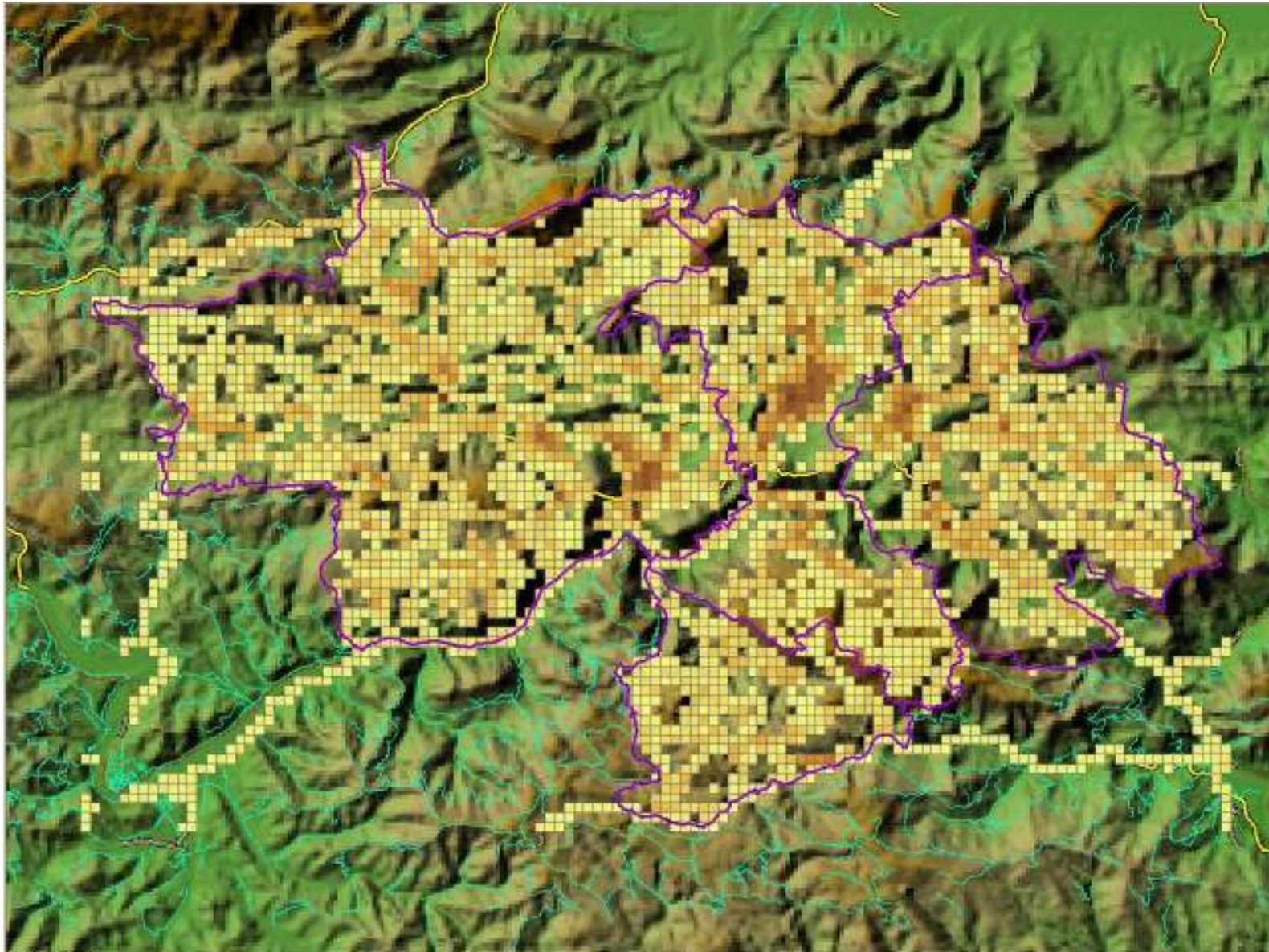
Slika P1.6: Karta skupnih emisij trdnih delcev TD v Zasavju v letu 2005.
