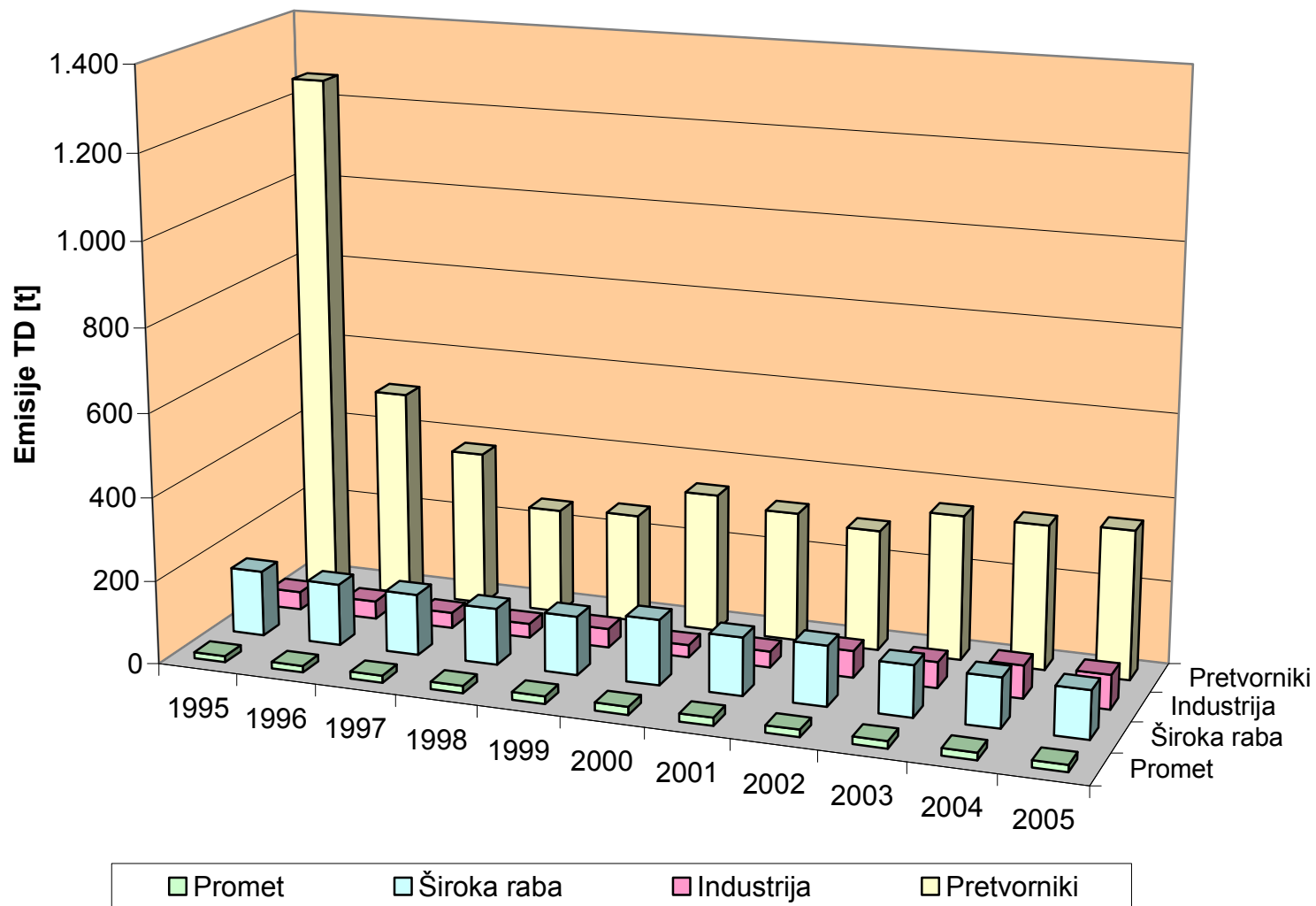
Slika P1.3: Ocena emisij trdnih delcev TD v Zasavju v obdobju 1995-2005.
