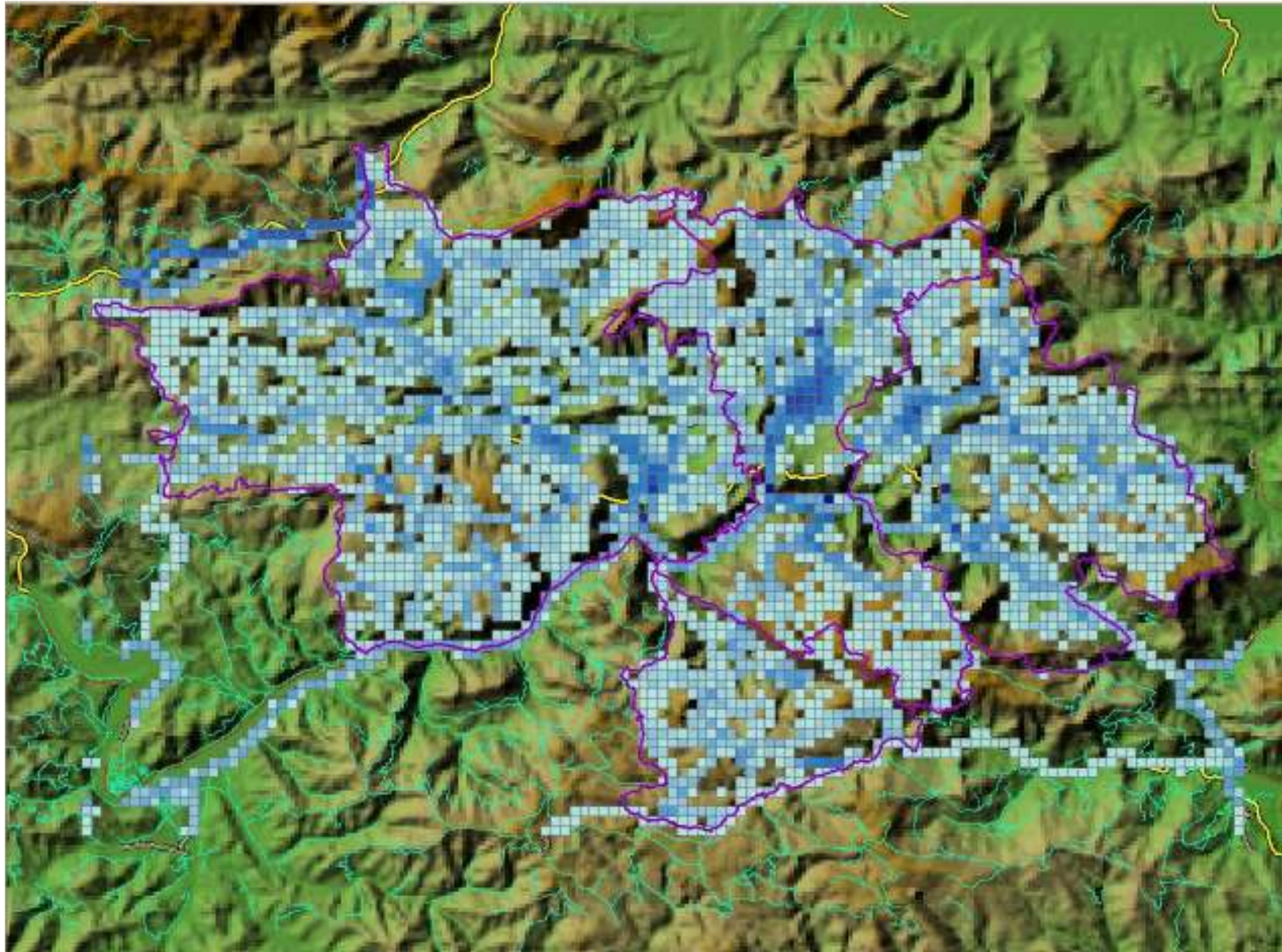
Slika P1.5: Karta skupnih emisij \text{NO}_x v Zasavju v letu 2005.
